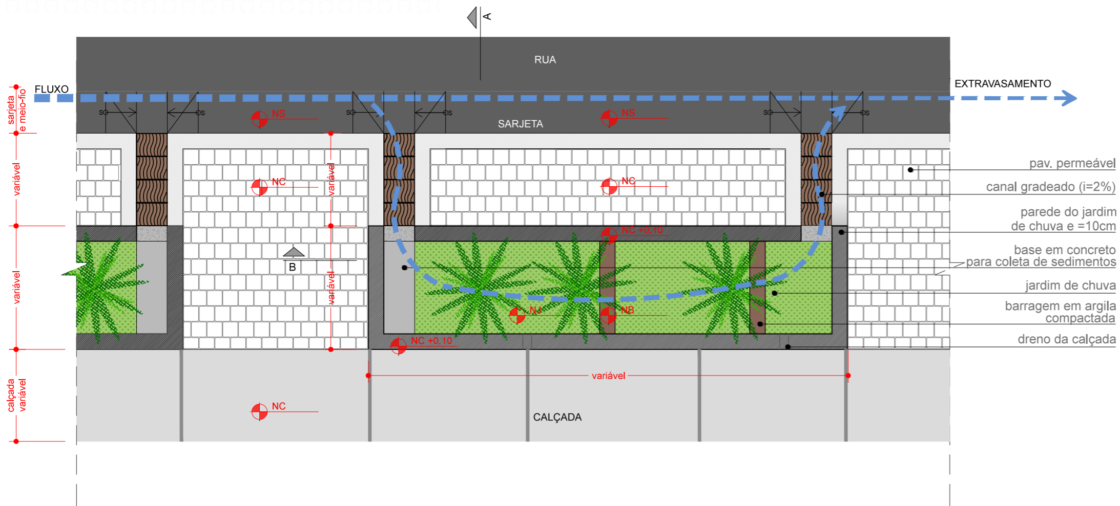
PLANTA
