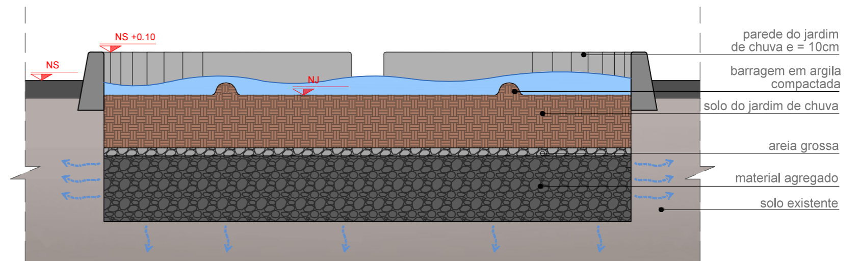
CORTE BB
