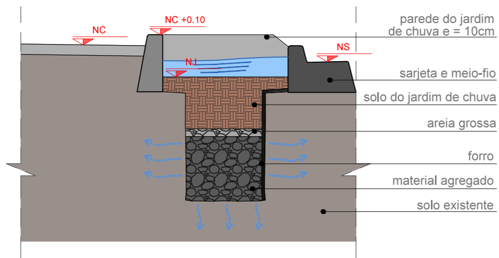
CORTE AA
