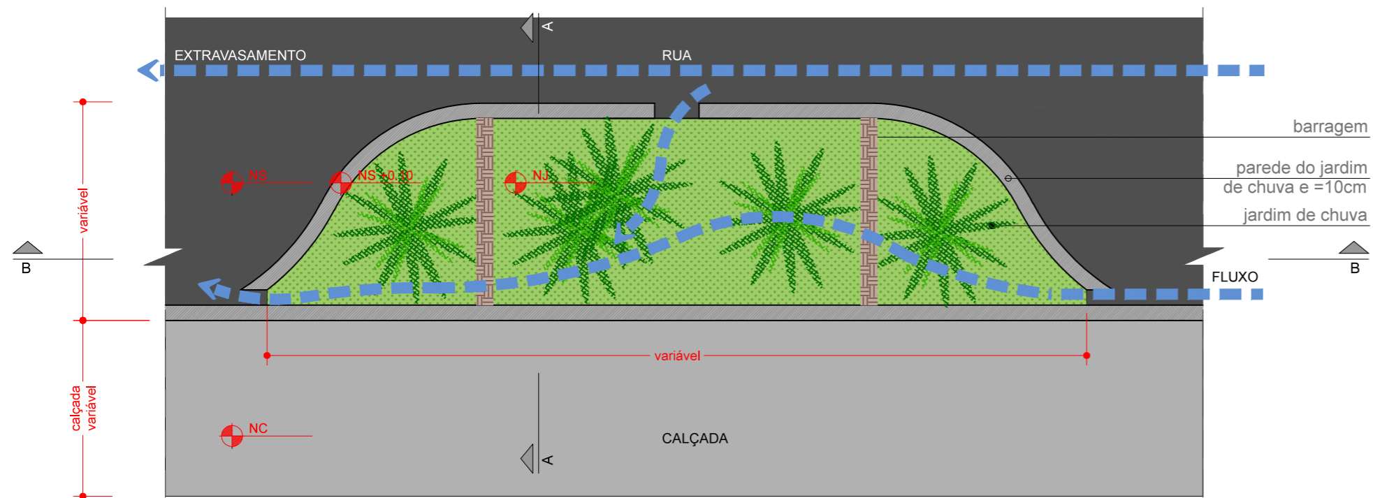
PLANTA
