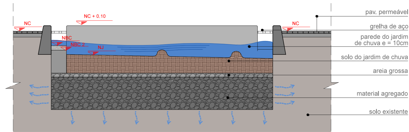
CORTE BB
